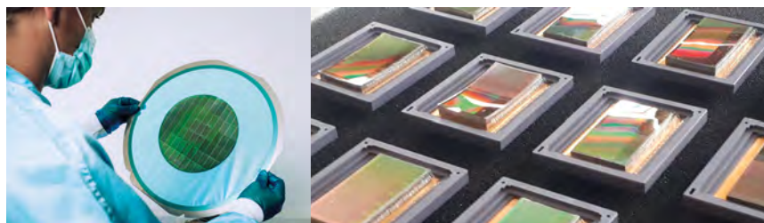
Figure 1. Capteurs courbes produits au Laboratoire d'Astrophysique de Marseille, basés sur la technologie de capteurs HDPYX de la société Pyxalis. Ces capteurs ont servi de démonstrateurs pour la mission de surveillance des aurores polaires depuis l'espace qui doit être opérationnelle en 2027.
