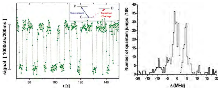
Figure 1. À gauche, « sauts quantiques » d'un ion unique (ici, un ion calcium) par absorption d'un photon vers le niveau métastable. Lorsque l'atome est dans le cycle de refroidissement, il fluoresce (niveau haut). Lorsque l'atome est dans le niveau métastable ("shelf"), il cesse de fluoresce pendant quelques secondes (niveau bas). À droite, statistique du nombre de sauts en fonction de la fréquence du laser excitant la transition d'horloge (laboratoire PIIM).
