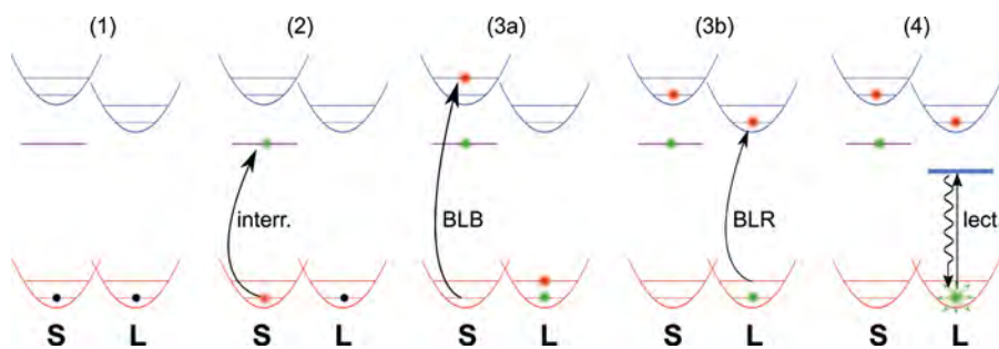
Figure 2. Étapes schématiques de la technique de spectroscopie par logique quantique. (1) Une paire d'ions est refroidie dans l'état fondamental d'un mode de vibration commun. Ce refroidissement se fait en agissant sur l'ion dit « logique » (L), l'ion d'intérêt spectroscopique (S) étant plus difficile à manipuler. (2) Un faisceau sonde « interroge » une transition très étroite de l'ion spectroscopique (transition d'horloge). En cas de succès l'électron passe dans le niveau excité (boule verte), sinon il reste dans l'état fondamental (boule rouge). (3) Comme il n'est pas possible de détecter directement l'état de l'ion S, on utilise l'état commun de vibration pour transférer cette information sur l'ion L. On effectue donc une tentative d'excitation de l'ion S sur une bande latérale bleue (BLB) d'une transition étroite auxiliaire (3a), suivie d'une tentative de « shelving » de l'ion L par une excitation de la bande latérale rouge (BLR, 3b). Ces deux étapes (3a et 3b) ne sont possibles que si l'ion S est resté dans l'état fondamental (boules rouges). (4) Une lecture de l'état de l'ion L révèle l'état initial de l'ion S. Les étapes élémentaires du transfert d'information entre ions via leur état commun de vibration (3a,3b) sont également à la base du fonctionnement de l'ordinateur quantique à ions piégés.
