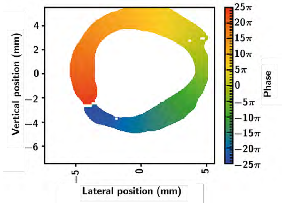
Figure 1. Image d'un analyseur de front d'onde Hartmann pour un faisceau vortex de l'harmonique 25 générée à partir d'un faisceau infrarouge portant un moment l=1 , reconstruction du profil d'intensité (à gauche) et du profil de phase (à droite).
