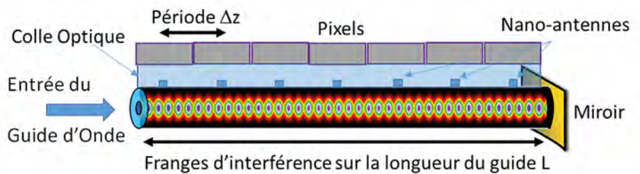
Figure 3. Concept du Spectromètre SWIFTS.
