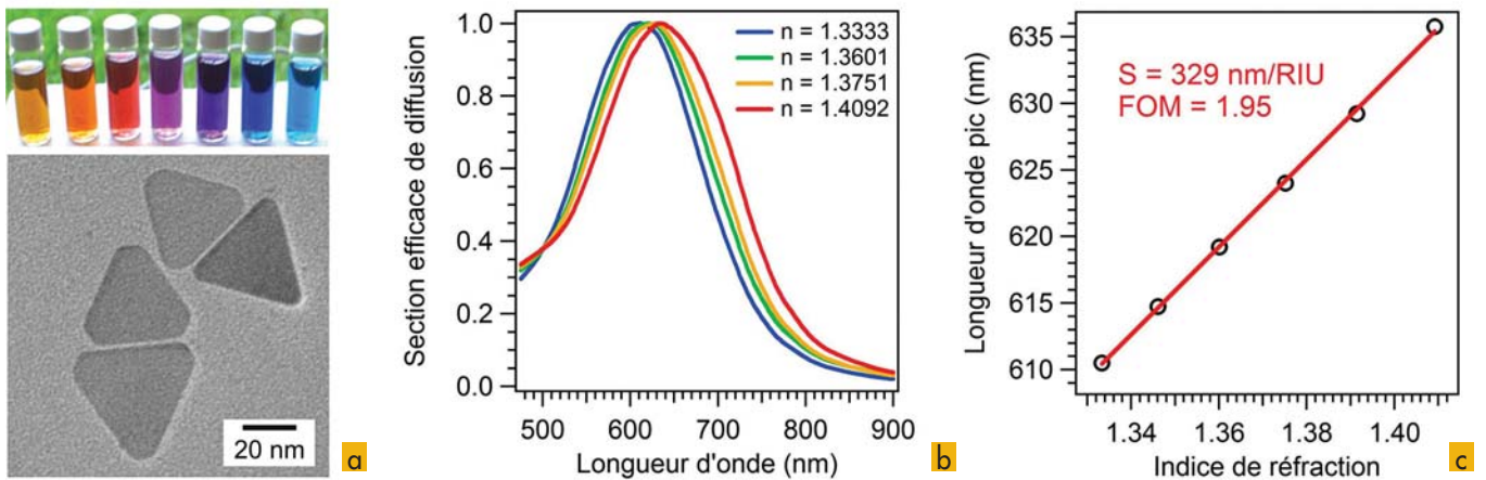
Figure 1. (a) Nanotriangles d'argent solubles dans l'eau, la taille des particules conditionne la longueur d'onde de résonance plasmon et donc la couleur de la solution. (b) Spectres de diffusion de nanotriangles d'argent dans différents mélanges eau-sucrose, une augmentation de l'indice de réfraction du milieu environnant les nanoparticules induit un décalage vers le rouge de la résonance plasmon. (c) Décalage en longueur d'onde de résonance en fonction de l'indice de réfraction du milieu. La pente de la courbe renseigne sur la sensibilité du système.
