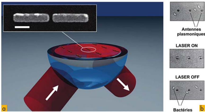
Figure 5. (a) Principe d'antennes optiques arrangées périodiquement sous illumination depuis le substrat de verre sous un angle de réflexion totale. (b) Série d'images successives montrant le piégeage de bactéries Escherichia coli lorsque l'illumination laser est présente. (Adapté avec la permission de [6].)
