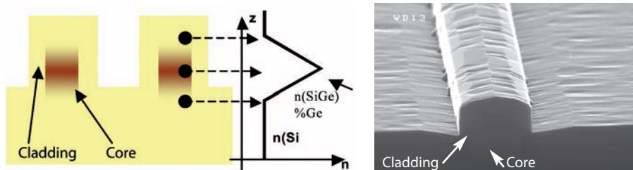
Figure 5. (a) Schéma du guide SiGe/Si à gradient de composition et (b) exemple de guide après fabrication.
