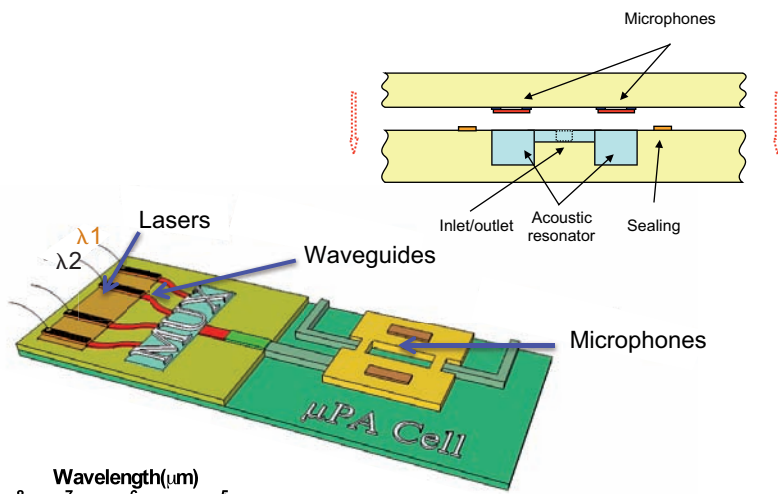
Figure 2. Capteur miniaturisé basé sur une source QCL multi-longueur d'onde accordable, un circuit photonique et un détecteur photoacoustique intégré sur la même puce de silicium.
