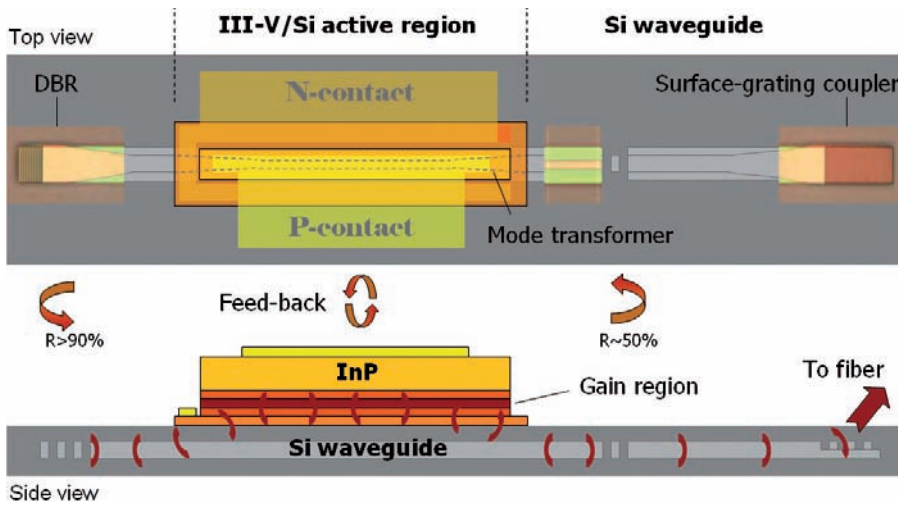
Figure 4. Exemple d'intégration hétérogène d'une source QCL sur guide Si [6].
